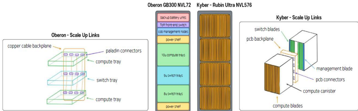
그림19 Oberon(GB200/300 NVL72) vs Kyber(Vera Rubin Ultra NVL 576 구조) 비교
