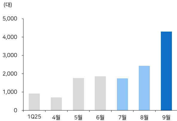
그림9 Nvidia GB200/GB300 NVL 72 서버랙 생산량 추이
