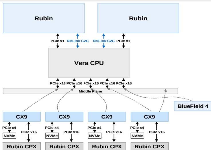
그림15 Vera Rubin NVL144 CPX Computing Tray 구조
