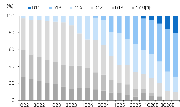
그림4 삼성전자 DRAM tech node 전망
